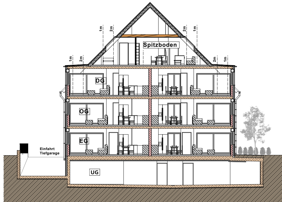
Schnitt B
